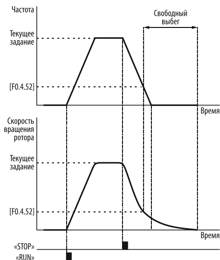
Рисунок 76 – обнаружение нулевой скорости при [F0.4.53] = «0» .
