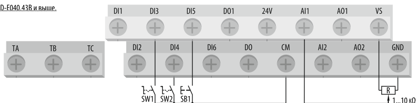
Рисунок 48 – схема подключения цепей управления при [F0.0.00] = «4» для AFD-E040.43B и выше.
