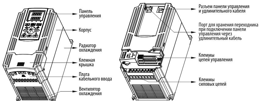
Рисунок 4 – тип корпуса 2, габариты 3, 4, 5 (модели AFD-E040.43B и выше)
