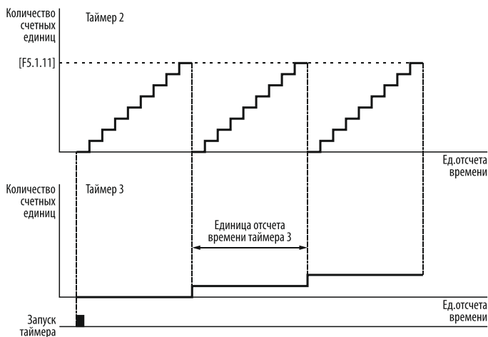
Рисунок 113 – единицы измерения таймеров 3 в завершённых циклах таймера 2.
