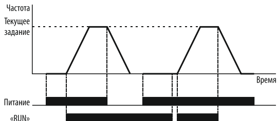
Рисунок 66 – автоматический запуск электродвигателя после включения питания «Запрещён».
