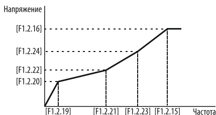
Рисунок 81 – пользовательская настройка U/f кривой.
