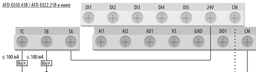
Рисунок 35 – схема подключения датчика с аналоговым выходным сигналом 0...10 В (питание от внешнего источника питания 24 В).
