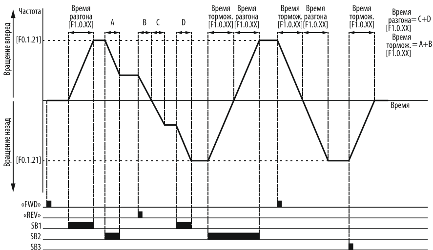
Рисунок 55 – двустороннее задание частоты с дискретных входов с возможностью управлением направлением вращения.
