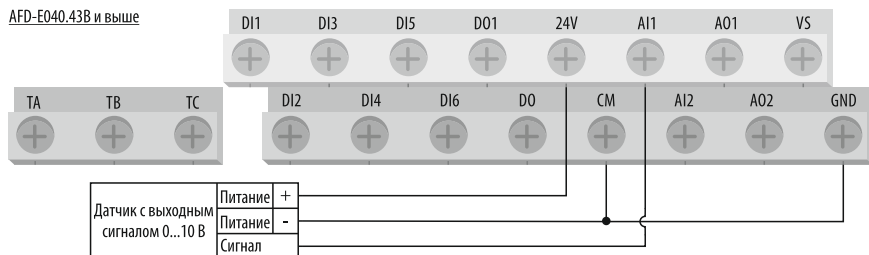
Рисунок 34 – схема подключения датчика с аналоговым выходным сигналом 0...10 В (питание от внутреннего источника питания 24 В).
