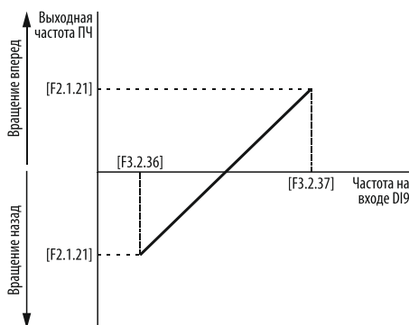
Рисунок 98 – масштабирование входного высокочастотного дискретного сигнала на высокоскоростном входе DI9 при [F0.2.25] = «15».
