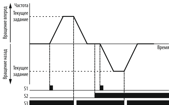
Рисунок 63 – трёхпроводной режим управления №2.
