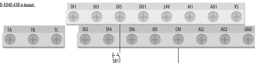
Рисунок 45 – схема подключения цепей управления при [F0.0.00] = «2» .
