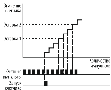
Рисунок 126 – счёт импульсов по заднему фронту импульсов.
