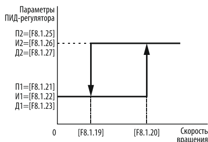
Рисунок 159 – переключение между ПИД1 и ПИД2 по гистерезису.
