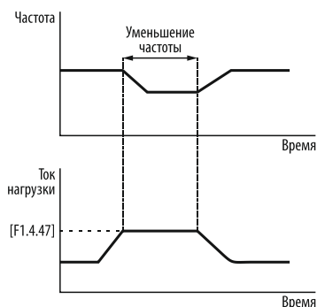
Рисунок 87 – Компенсация повышения тока нагрузки.
