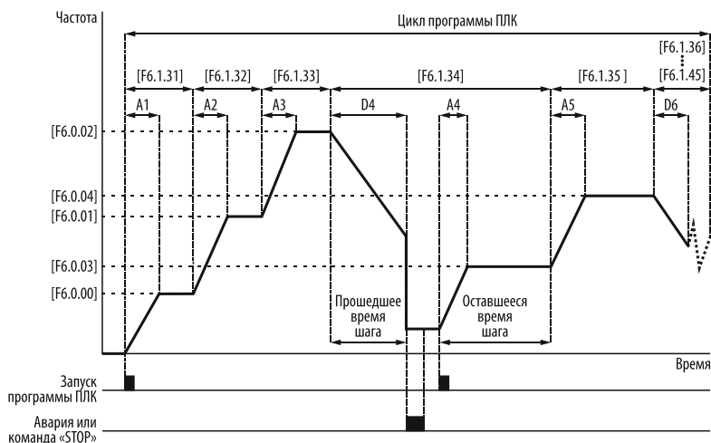
Рисунок 148 – запуск программы ПЛК с частоты шага прерывания программы.
