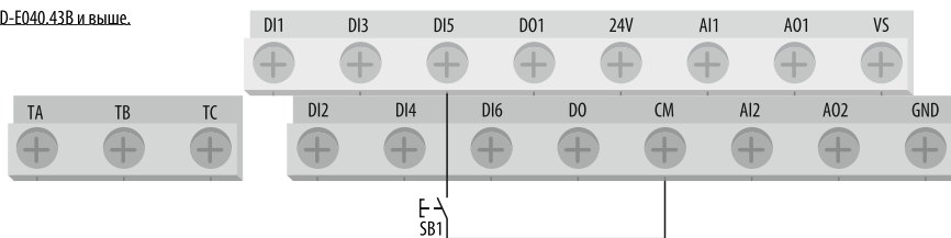
Рисунок 44 – схема подключения цепей управления при [F0.0.00] = «1» для AFD-E040.43B и выше.
