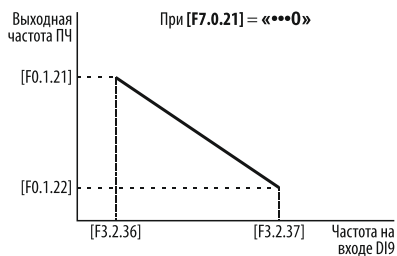
Рисунок 99 – масштабирование входного высокочастотного дискретного сигнала на высокоскоростном входе DI9 при или [F7.0.10] = «4».
