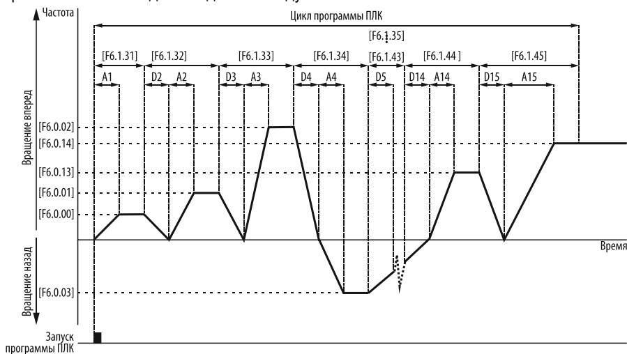
Рисунок 146 – один цикл с остановкой между шагами и работой на частоте последнего шага по окончании цикла.
