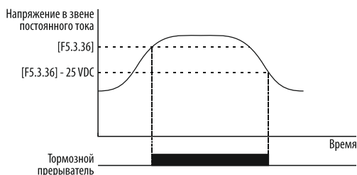
Рисунок 139 – диапазон напряжения в звене постоянного тока для включения / отключения тормозного прерывателя.
