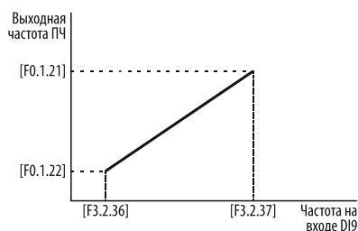
Рисунок 97 – масштабирование входного высокочастотного дискретного сигнала на высокоскоростном входе DI9 при [F0.2.25] = «14».
