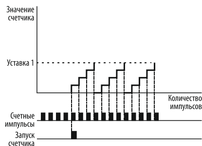
Рисунок 133— сброс текущего значения счётчика по достижении уставки 1.
