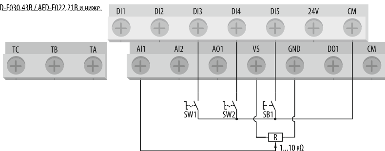
Рисунок 47 – схема подключения цепей управления при [F0.0.00] = «4» для AFD-E030.43B / AFD-E022.21B и ниже.
