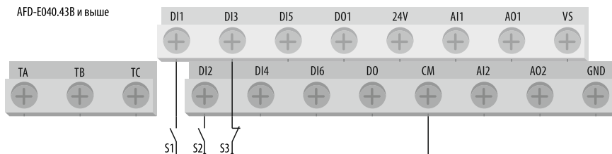
Рисунок 64 – подключение внешних управляющих сигналов при трёхпроводном режиме управления №1 и №2.
