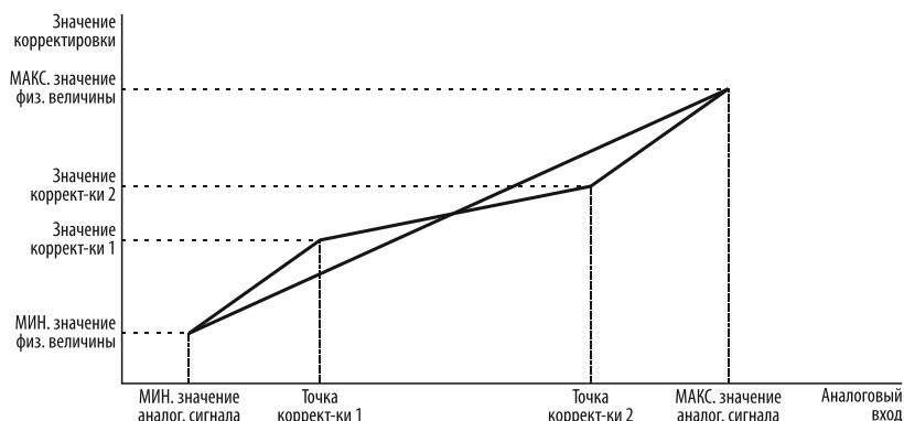
Рисунок 107 – корректировка кривой аналоговых входов AI1 , AI2 , AI3 .
