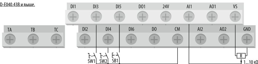
Рисунок 46 – схема подключения цепей управления при [F0.0.00] = «3» .
