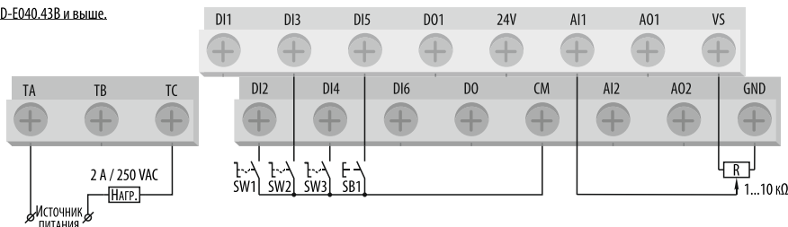
Рисунок 50 – схема подключения цепей управления при [F0.0.00] = «6».
