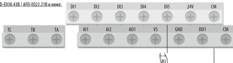
Рисунок 43 – схема подключения цепей управления при [F0.0.00] = «1» для AFD-E030.43B / AFD-E022.21B и ниже.
