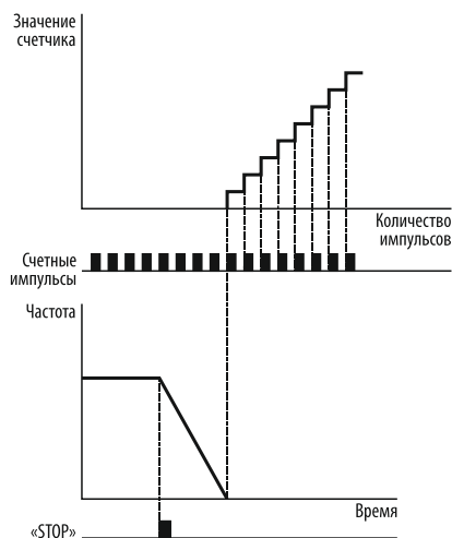
Рисунок 131 – запуск счётчика при остановке электродвигателя.
