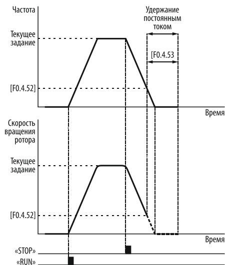
Рисунок 77 – обнаружение нулевой скорости при [F0.4.53] \neq «0» .
