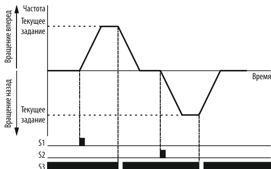
Рисунок 62 – трёхпроводной режим управления №1.
