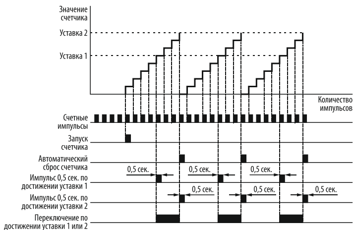
Рисунок 137– автоматический сброс текущего значения счётчика по достижении уставки 2.
