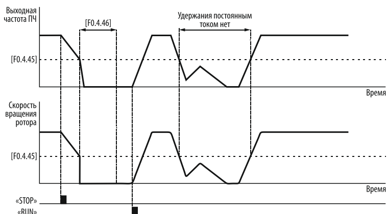
Рисунок 71 – удержание постоянным током при команде «STOP».
