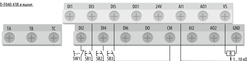
Рисунок 49 – Схема подключения цепей управления при [F0.0.00] = «5»
