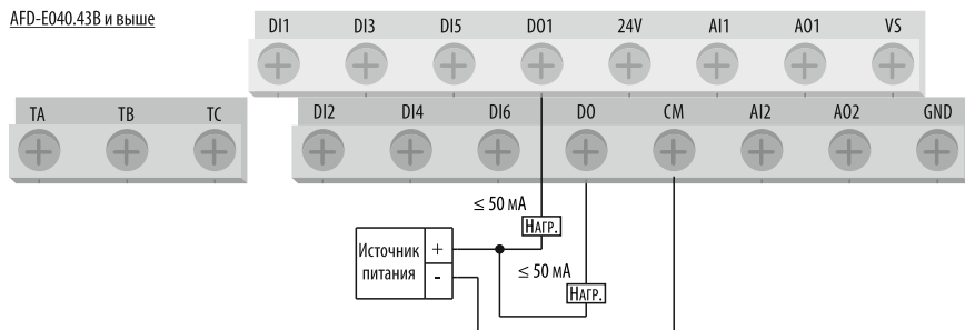
Рисунок 39 – схема подключения нагрузки к транзисторному выходу (питание от внешнего источника питания 24 В).
