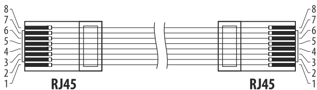
Рисунок 40 – схема кабеля для подключения панели управления к ПЧ при выносном монтаже. (Тип кабеля: экранированный сетевой кабель Cat.5е, тип разъёма: RJ-45, разводка: TIA / EIA-T568B.
