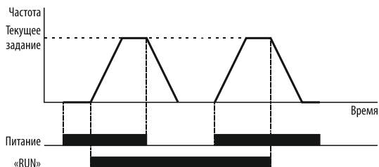
Рисунок 65 – автоматический запуск электродвигателя после включения питания «Разрешён».
