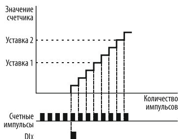
Рисунок 129 – запуск счётчика по сигналу на дискретном входе.
