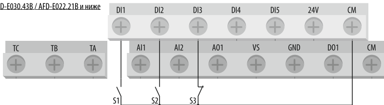
Рисунок 63 – трёхпроводной режим управления №2.
