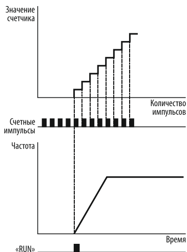
Рисунок 130 – запуск счётчика при запуске электродвигателя.
