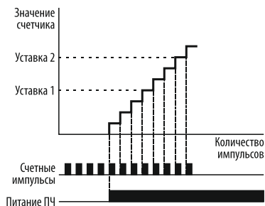
Рисунок 128 – запуск счётчика при подаче питания ПЧ.
