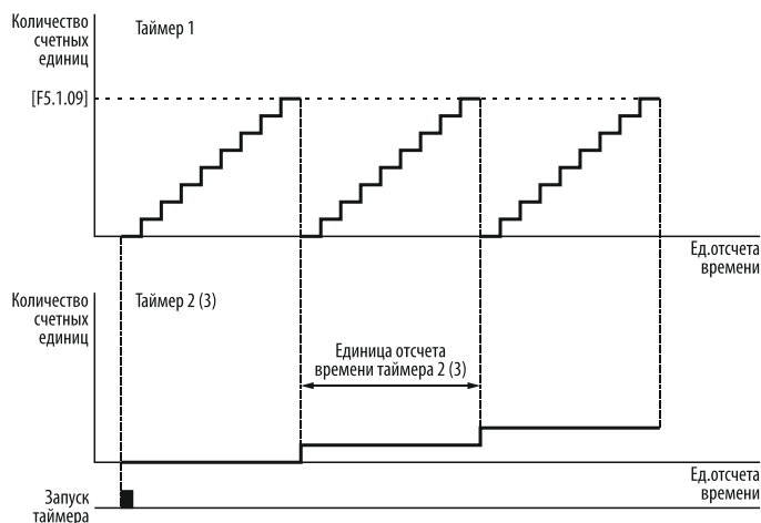
Рисунок 112 – единицы измерения таймеров 2 и 3 в завершённых циклах таймера 1.
