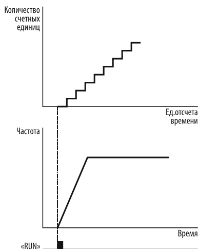
Рисунок 115 – запуск таймера при запуске электродвигателя.
