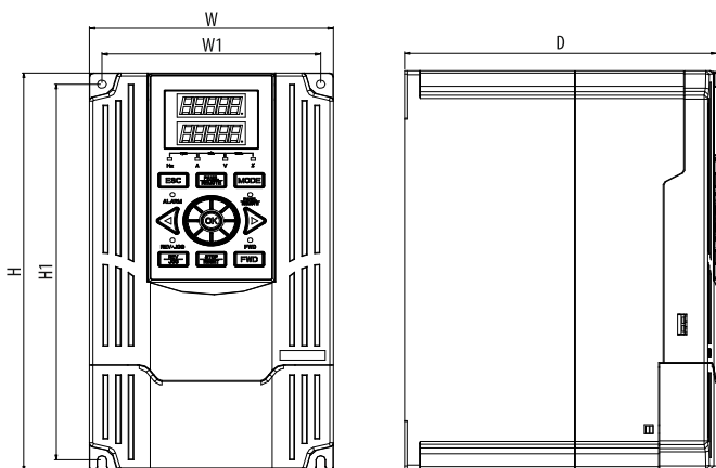
Рисунок 12 – габаритные размеры AFD-E040.43B и выше (тип корпуса 2, габариты 3, 4, 5)
