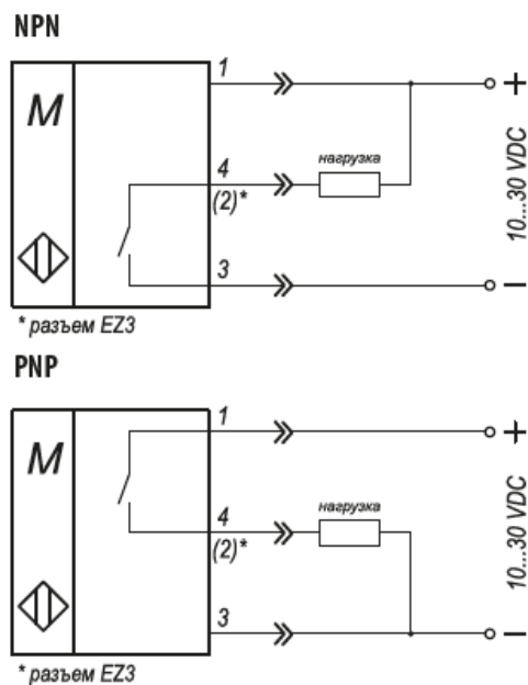
Рисунок 5 – Схемы подключения трехпроводных NO датчиков LM50-34.11.U1.K08, LM50-34.11.U1.KZ3
