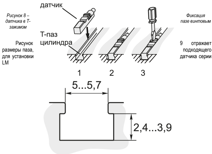
Рисунок 9 – Размеры Т-паза пневмоцилиндра для датчиков серии LM
