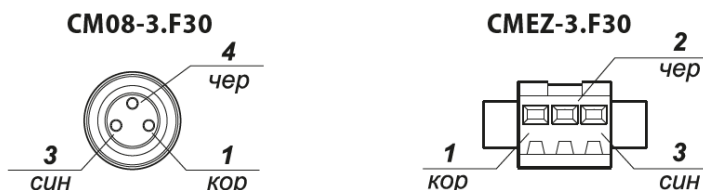
Рисунок 12 – Распиновка соединителей KIPPRIBOR серии CM
